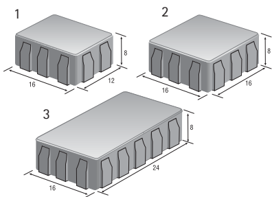
Beispiele Verlegemuster
